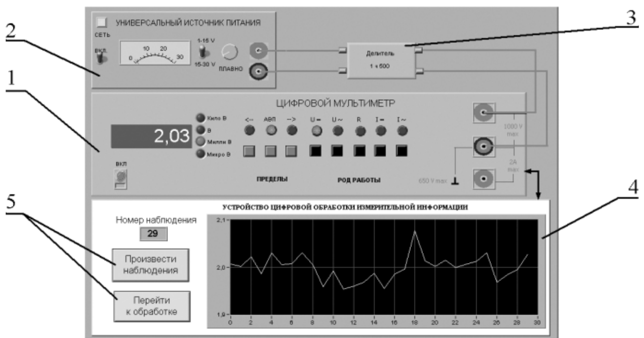
Рис. 1.4.1. Вид модели лабораторного стенда на рабочем столе компьютера при выполнении лабораторной работы №1.4 (1-электронный цифровой мультиметр, 2-универсальный источник питания, 3-делитель напряжения, 4-индикатор устройства обработки измерительной информации, 5-элементы управления устройством обработки измерительной информации).
